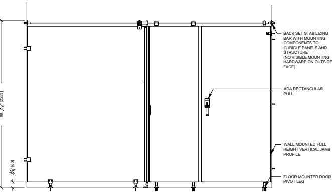
B-B ELEVATION
