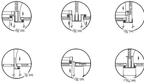
JAMB PROFILES
