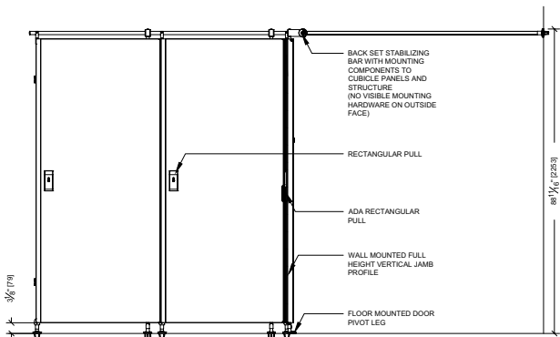
A-A ELEVATION
